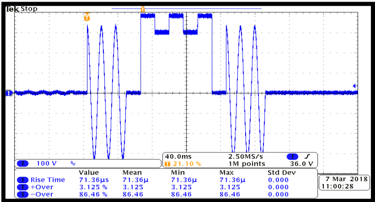
Actual output voltage waveform
