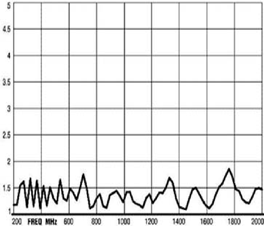
3148B Log Periodic Dipole Array Antenna VSWR
